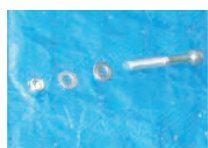
VITE M8x40 TCEI ZN ROSETA 8.4x16 H1.6 ZN TUERCA AUTOBL. M8 ZN
